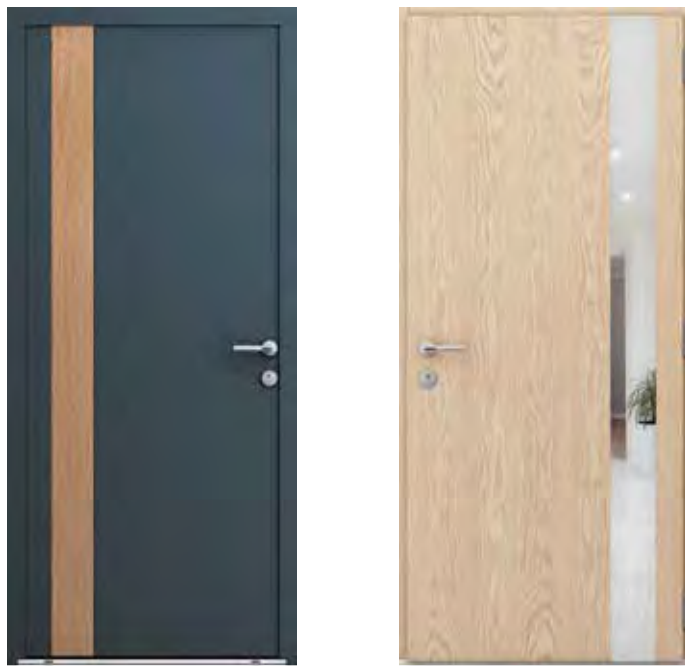
EXTÉRIEUR ALUMINIUM Couleur gris 7016 T. Insert décor ton bois. INTÉRIEUR BOIS Finition chêne champagne. Insert décor miroir. Ud ≥ 0,7 W/m².K
